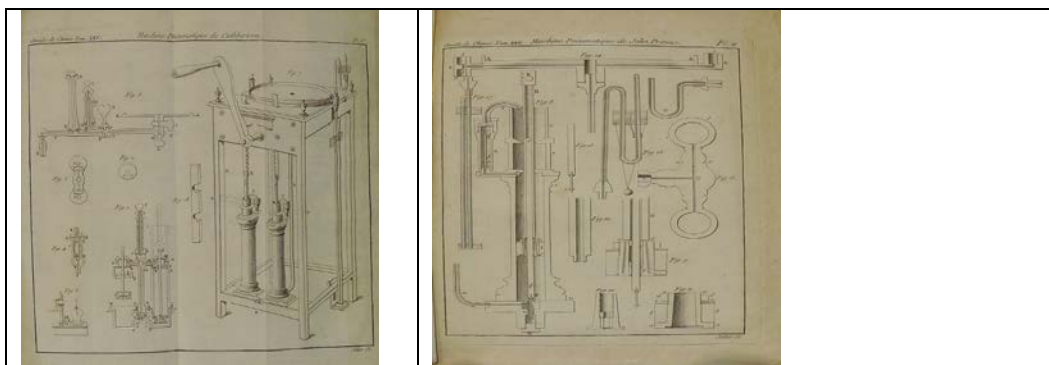
Fig. 2. Sinistra: tavola tratta dagli Annali di Chimica (Adet 1798) in cui in Fig. 7 è rappresentata la Pompa di Cathbertson nel suo insieme. Destra: Nella tavola tratta dallo stesso testo sono rappresentati i particolari della pompa
