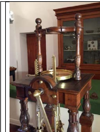
Fig. 5. Sinistra: particolare del telaio sul ripiano superiore che deve trattenere saldamente il recipiente quando la pompa comprime l'aria al suo interno. Destra: rubinetto a due vie che apre la comunicazione con il tubo lungo (la pompa rarefa l'aria) o con il tubo corto (la pompa comprime l'aria)
