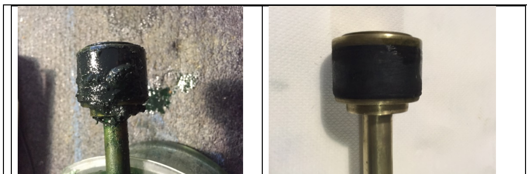
Fig. 6. Uno dei pistoni prima della pulizia (sinistra) e dopo (destra)
